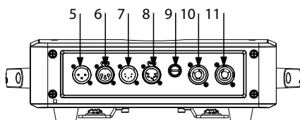
Pannello B
