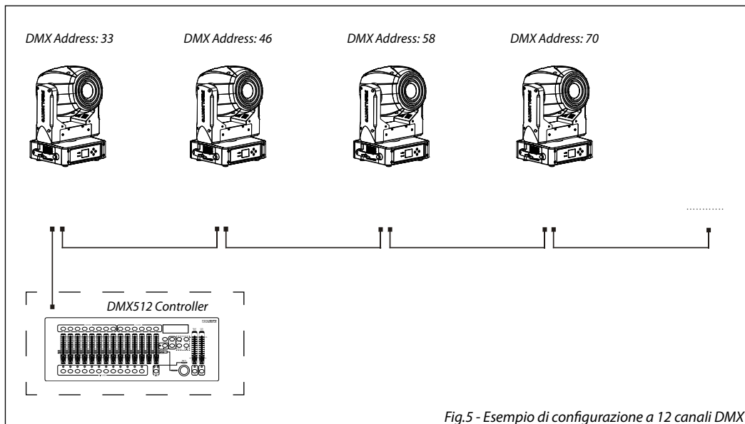
Fig.5 - Esempio di configurazione a 12 canali DMX
